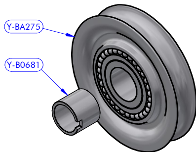
Code 10021A Sheave assy D100 - 020 L21 AL Black (OPF 100)
