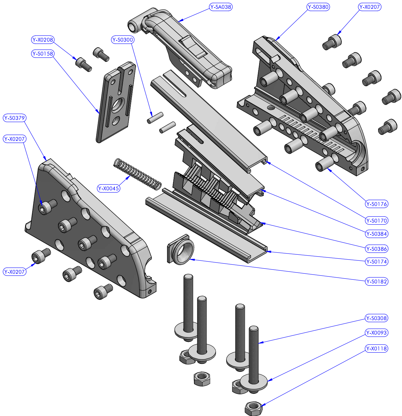
Cod.Y-SA038 Lever assy
