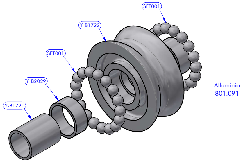
ELENCO PARTI 801.091
